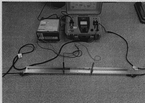
(a) 시료 #1 시험전경
